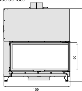
Plan d'ensemble
