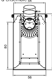
Plan d'ensemble 54
