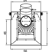
Plan d'ensemble
