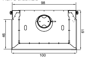
Plan d'ensemble
