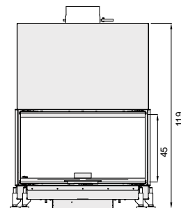
Plan d'ensemble
