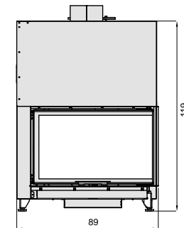
Plan d'ensemble
