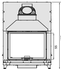
Plan d'ensemble
