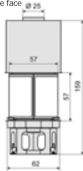
Plan d'ensemble
