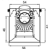
Plan d'ensemble
