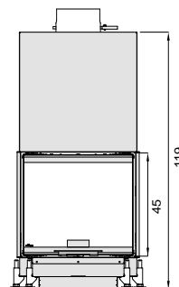
Plan d'ensemble 54
