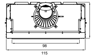
Plan d'ensemble
