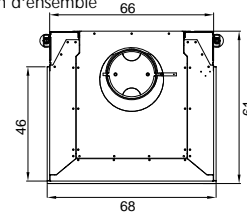
Plan d'ensemble
