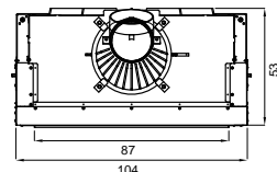
Plan d'ensemble
