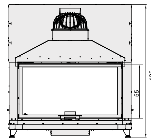
Plan d'ensemble
