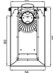
Plan d'ensemble 54
