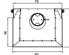
Plan d'ensemble
