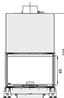
Plan d'ensemble
