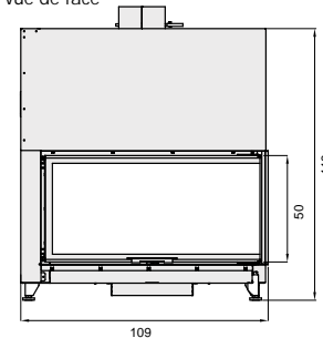
Plan d'ensemble
