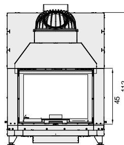
Plan d'ensemble
