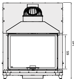
Plan d'ensemble
