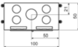
Plan d'ensemble
