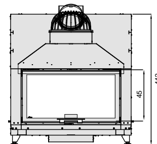
Plan d'ensemble
