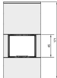
Plan d'ensemble
