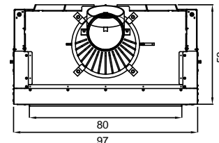
Plan d'ensemble
