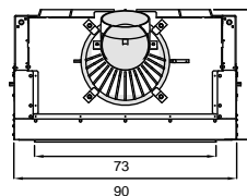
Plan d'ensemble
