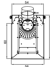
Plan d'ensemble
