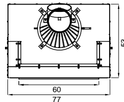
Plan d'ensemble
