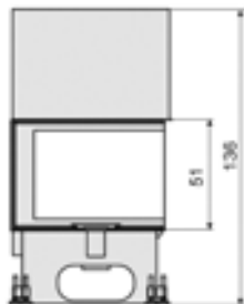
Plan d'ensemble
