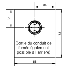
Plan d'ensemble
