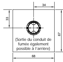
Plan d'ensemble
